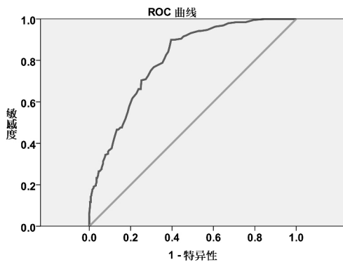
图 2 二元 Logistic 回归预测优秀提案概率的 ROC 曲线
