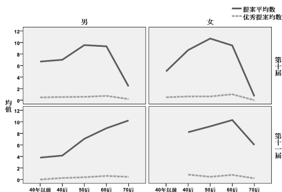
图1 年龄分层和性别对提案总数及优秀提案数影响的多重线图
